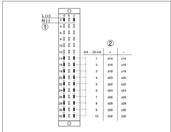
Abb. 3: VEGALOG 571 AA 1)
