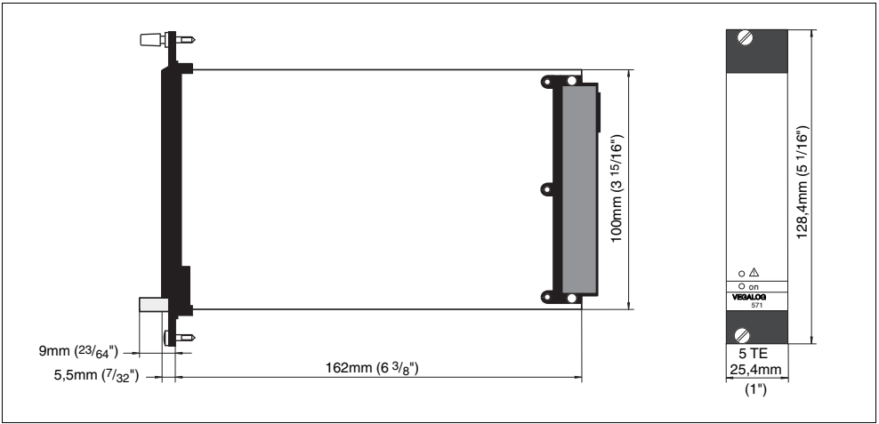
Abb. 5: Maße VEGALOG 571 AA
