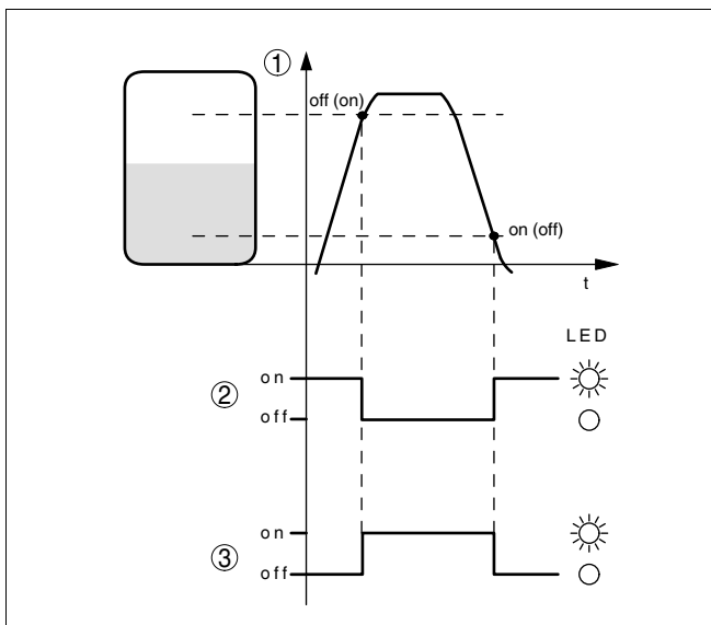
Рис. 8: Режимы работы реле
