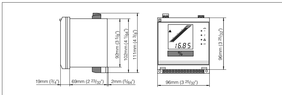
Рис. 9: Размеры VEGAMET 381 Ex
