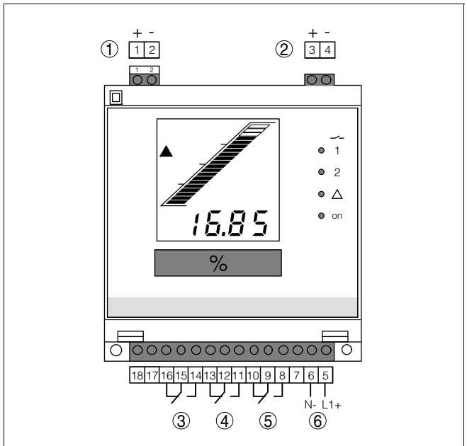
Рис. 6: Схема расположения контактов VEGAMET 381 Ex 1 Вход данных измерения/питание датчика с гнездом для VEGACONNECT 2 Токовый выход 3 Реле сигнала неисправности 4 Реле 2 5 Реле 1 6 Питание
