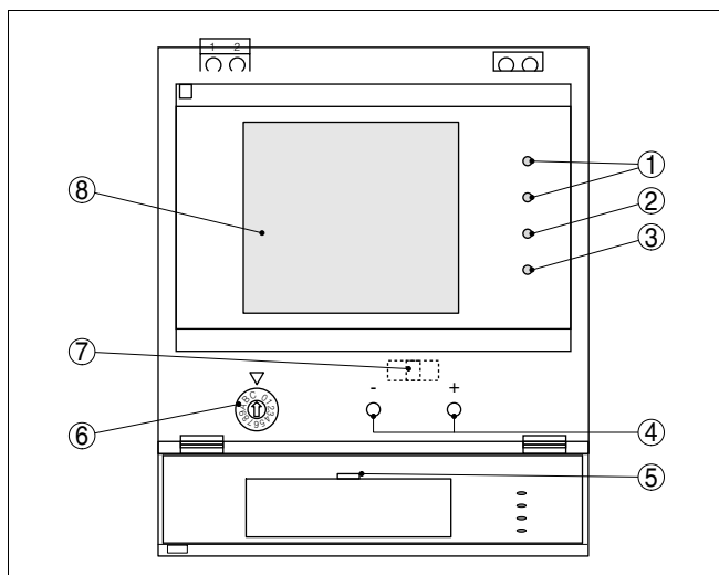
Рис. 1: VEGAMET 381 Ex
